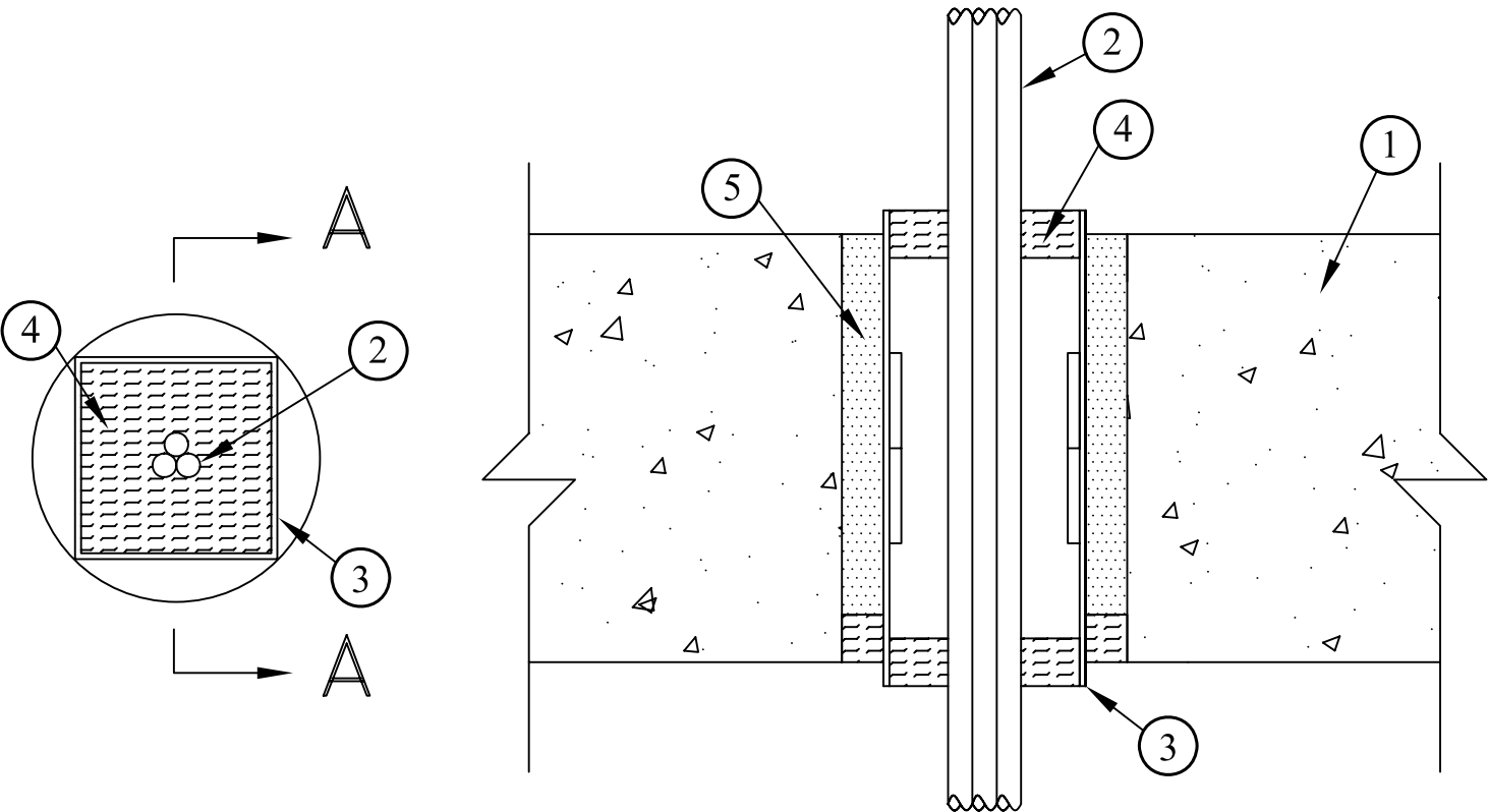
SECTION A-A
